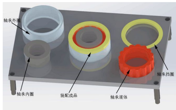
图 13 装配参考图
